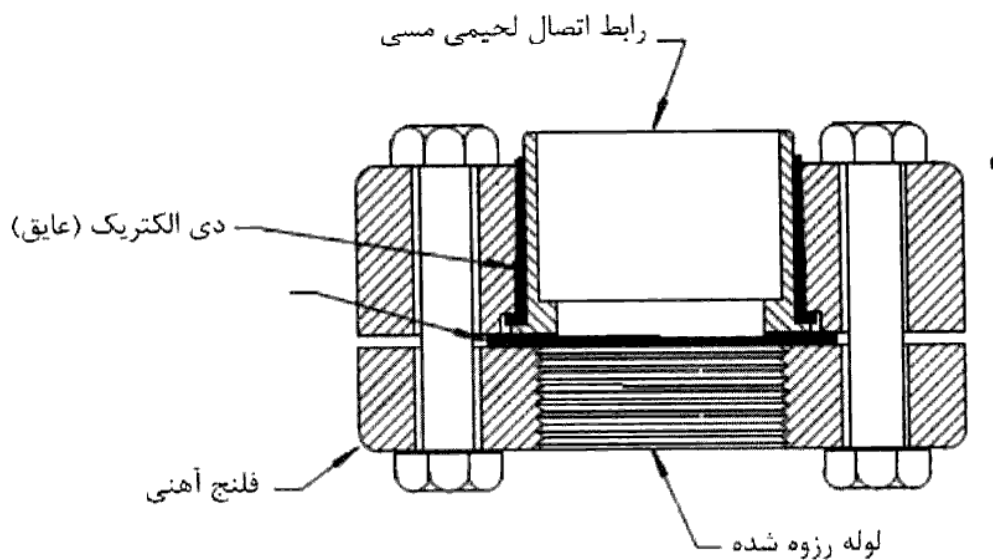
شکل (۱۲-۴-۱۶) وصاله فلنجی دی الکتریک
