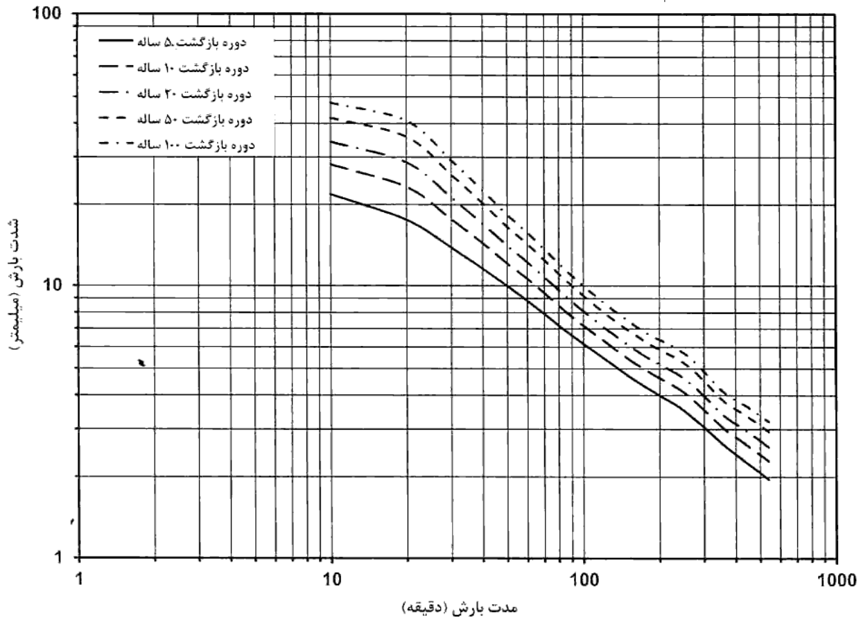
شکل شماره (۱۶-۸-۳) نمودار شدت-مدت- فراوانی بارندگی برای ایستگاه سینوپتیک مهرآباد تهران
