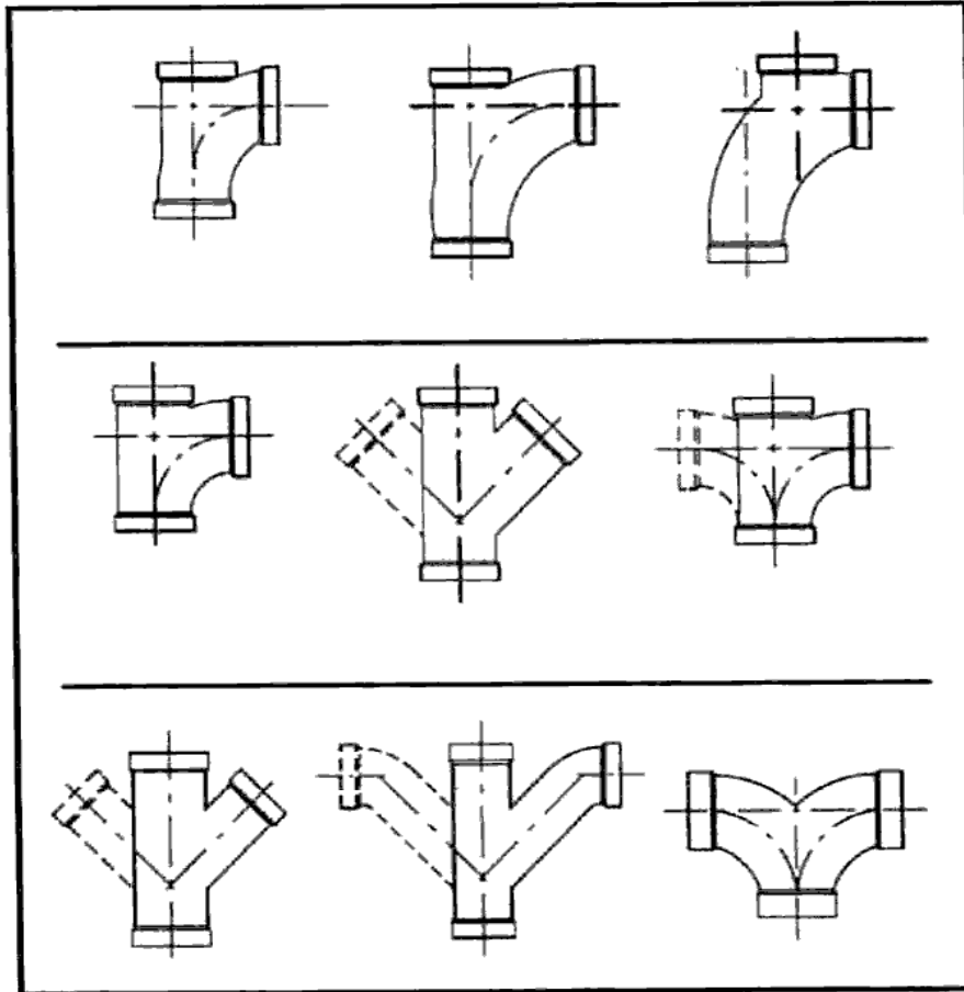
شکل (۳۶-۵-۳۸) انواع وصاله‌های قابل استفاده در شبکه فاضلاب
