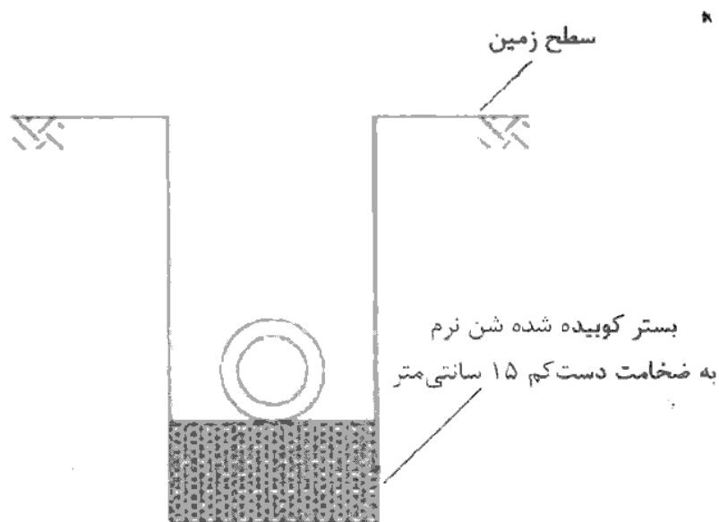
شکل (۱۶-۲-۹) ترنج (کانال) حفاری شده برای لوله گذاری
