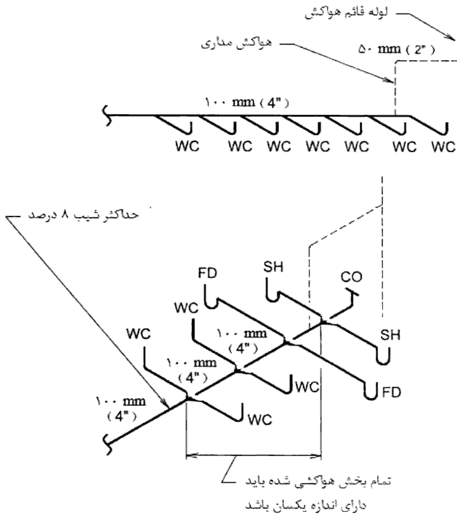
شکل شماره (۱۶-۶-۳۰) اندازه‌گذاری هواکش مداری
