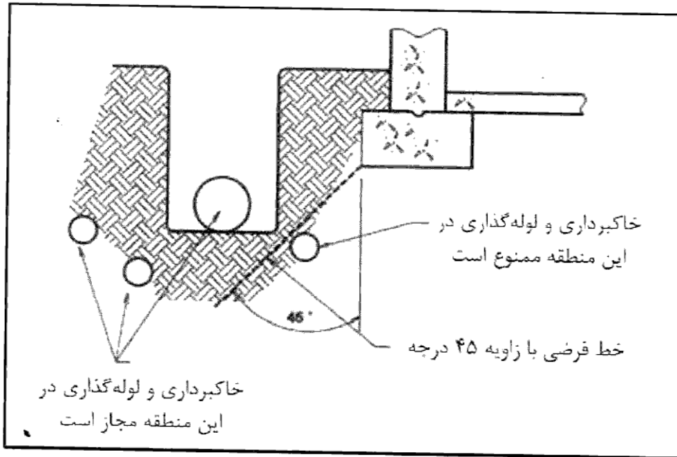
شکل (۱۶-۵-۴۱) الزامات حفاری و لوله گذاری زیر پی ساختمان
