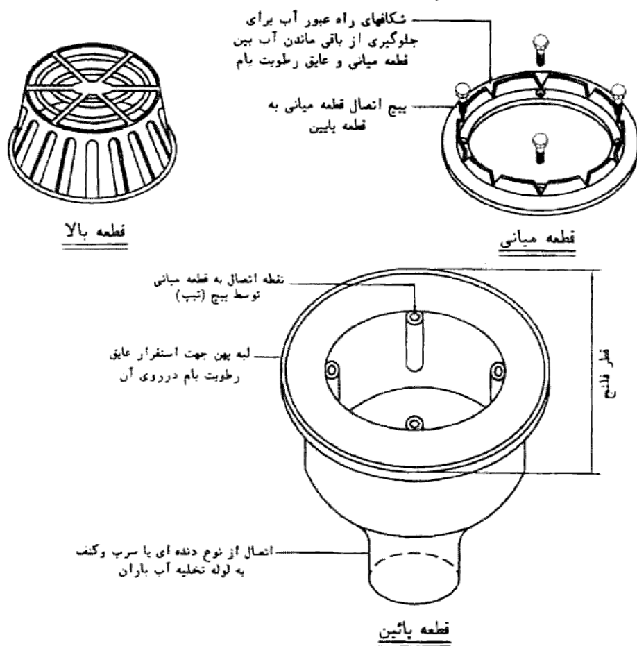
شکل شماره (۴-۸-۱۶) قطعات کفشوی آب باران
