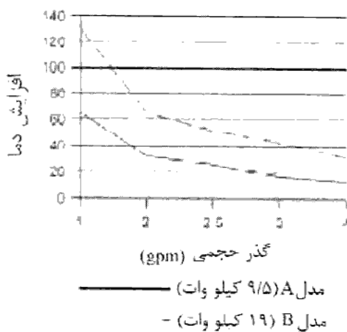
شکل (۱۶-۴-۴۷) نمودار ظرفیت آب گرم کن فوری
