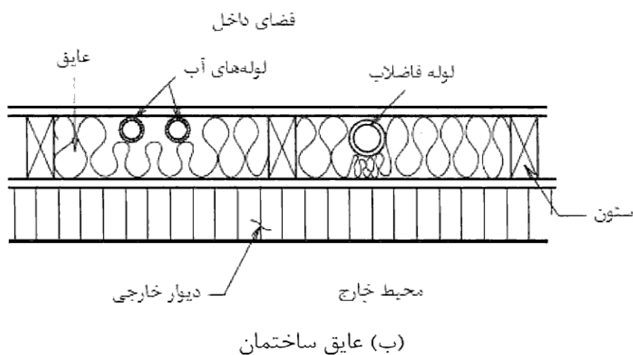
شکل (۳-۱۶-۴) حفاظت از لوله در برابر یخ‌زدگی
