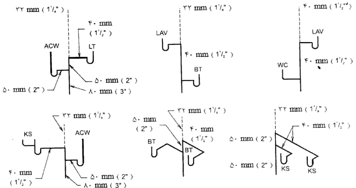
شکل شماره (۱۵-۶-۱۶) هواکش مشترک برای وسایل بهداشتی در طبقات مختلف
