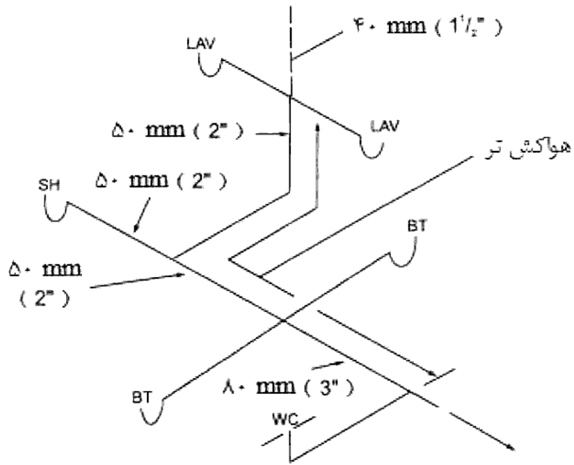
شکل شماره (۱۶-۶-۲۱) هواکش تر برای حمام‌های مجاور
