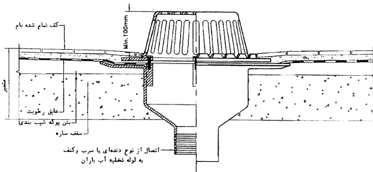
شکل شماره (۵-۸-۱۶) جزئیات نصب کفشوی آب باران با کلاهک مشبک
