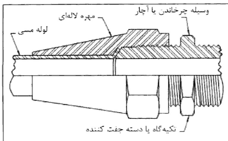
شکل (۱۶-۴-۸) یک اتصال وصله فشاری
