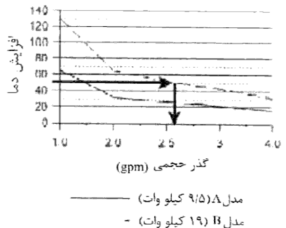
شکل (۱۶-۴-۴۸) نقطه عملکرد آب گرم کن فوری
