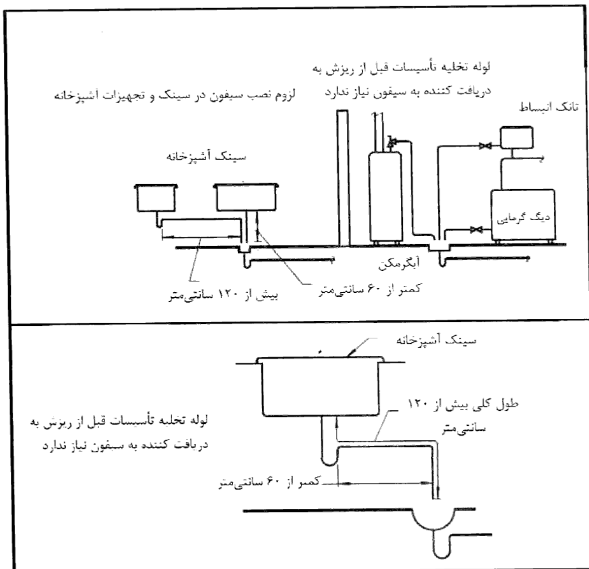
شکل (۱۶-۵-۲۷) نیاز/عدم نیاز نصب سیفون بر روی لوله تخلیه تأسیسات با اتصال
