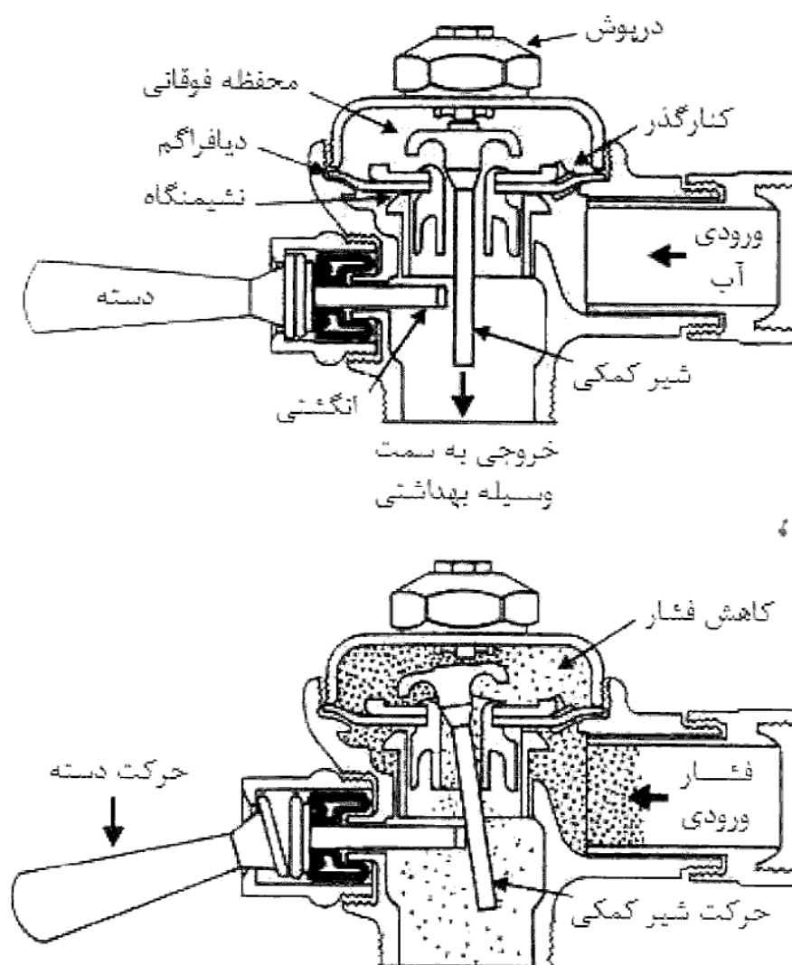
شکل شماره (۱۶-۷-۹) نحوه عملکرد فلاش والو دیافراگمی
