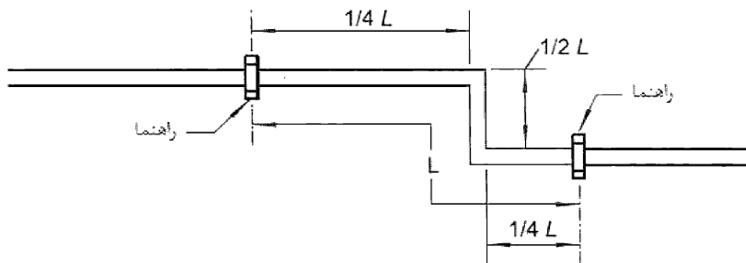
(ب) خم Z شکل
