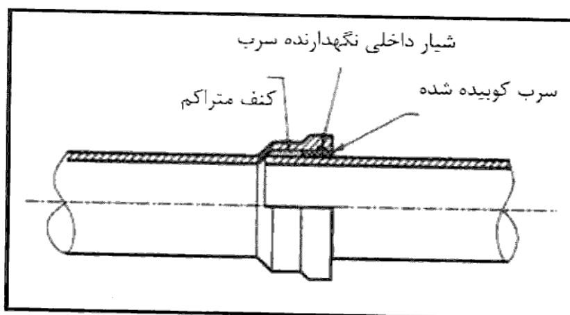
شکل (۱۶-۵-۴۴) اتصال با سرب و کنف لوله چدنی سرکاسه‌دار
