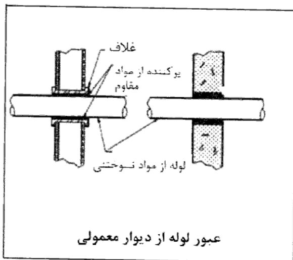
شکل (۱۶-۵-۴۲) جزئیات عبور لوله از دیوار
