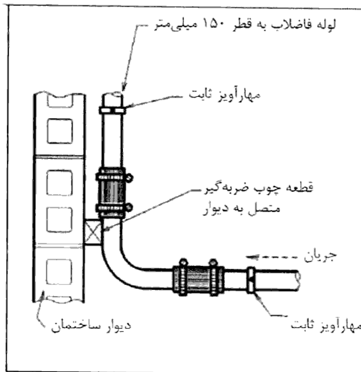
شکل (۴-۹-۱۶) جزئیات مهارسازی قطعات انبساط‌گیر روی لوله فاضلاب
