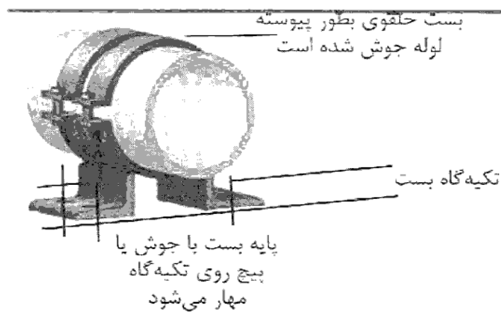
شکل (۱۶-۲-۲۳) نمونه‌ای از مه‌ار لوله
