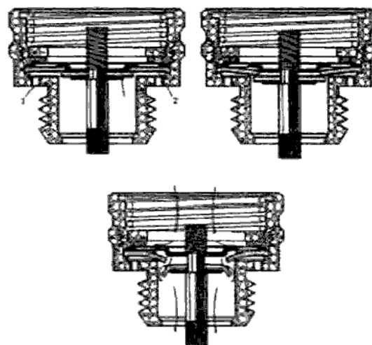
شکل (۱۶-۴-۴۲) خلاءشکن اتصال سرشلنگی شکل (۱۶-۴-۴۱) شیر سرشلنگی ضدیخ با تجهیزات داخلی ضدسیفون
