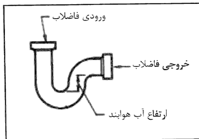
شکل (۱۶-۲-۱۵) عمق آب هوا بند سیفون
