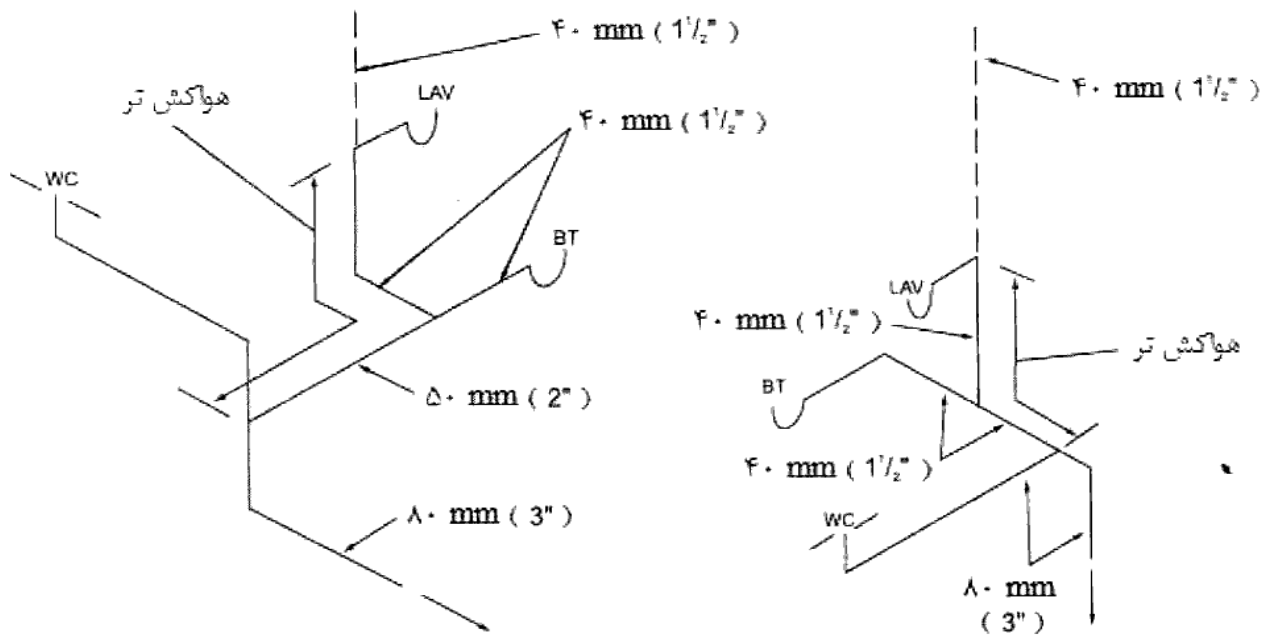
شکل شماره (۱۶-۶-۲۲) دو نمونه دیگر از هواکش تر
