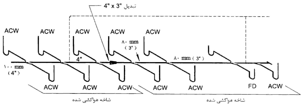
شکل شماره (۱۶-۶-۳۱) تغییر اندازه لوله در هواکش مداری
