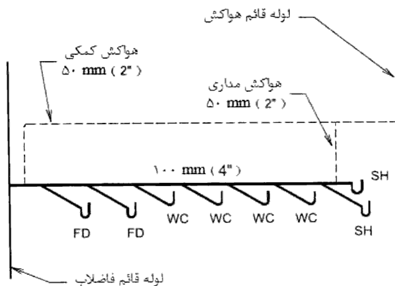
شکل شماره (۱۶-۶-۳۲) هواکش کمکی
