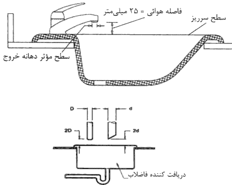
شکل (۱۶-۲-۲۰) فاصله هوایی
