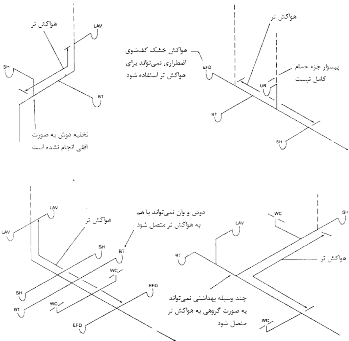
شکل شماره (۱۶-۶-۲۴) نمونه‌هایی از استفاده نادرست از هواکش تر (قسمت دوم)
