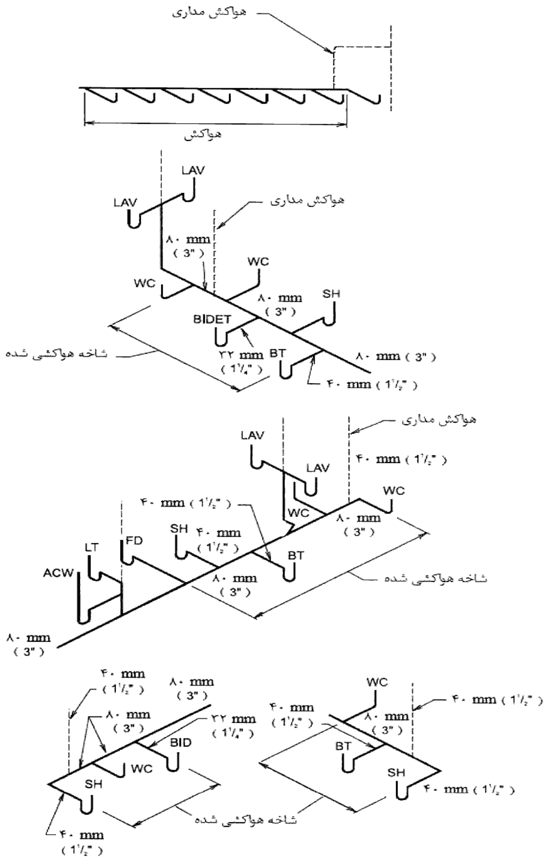
شکل شماره (۱۶-۶-۲۷) هواکش مناری
