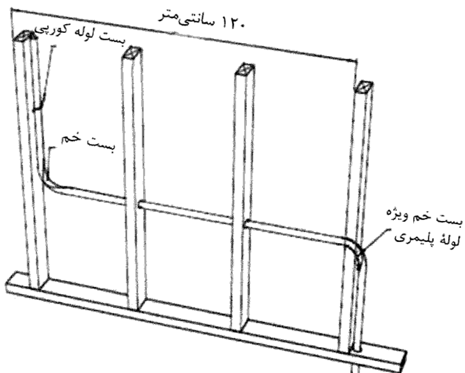
شکل (۱۰-۹-۱۶) استفاده از بست مخصوص خم در نقطه انتهایی تبدیل لوله قائم به لوله افقی
