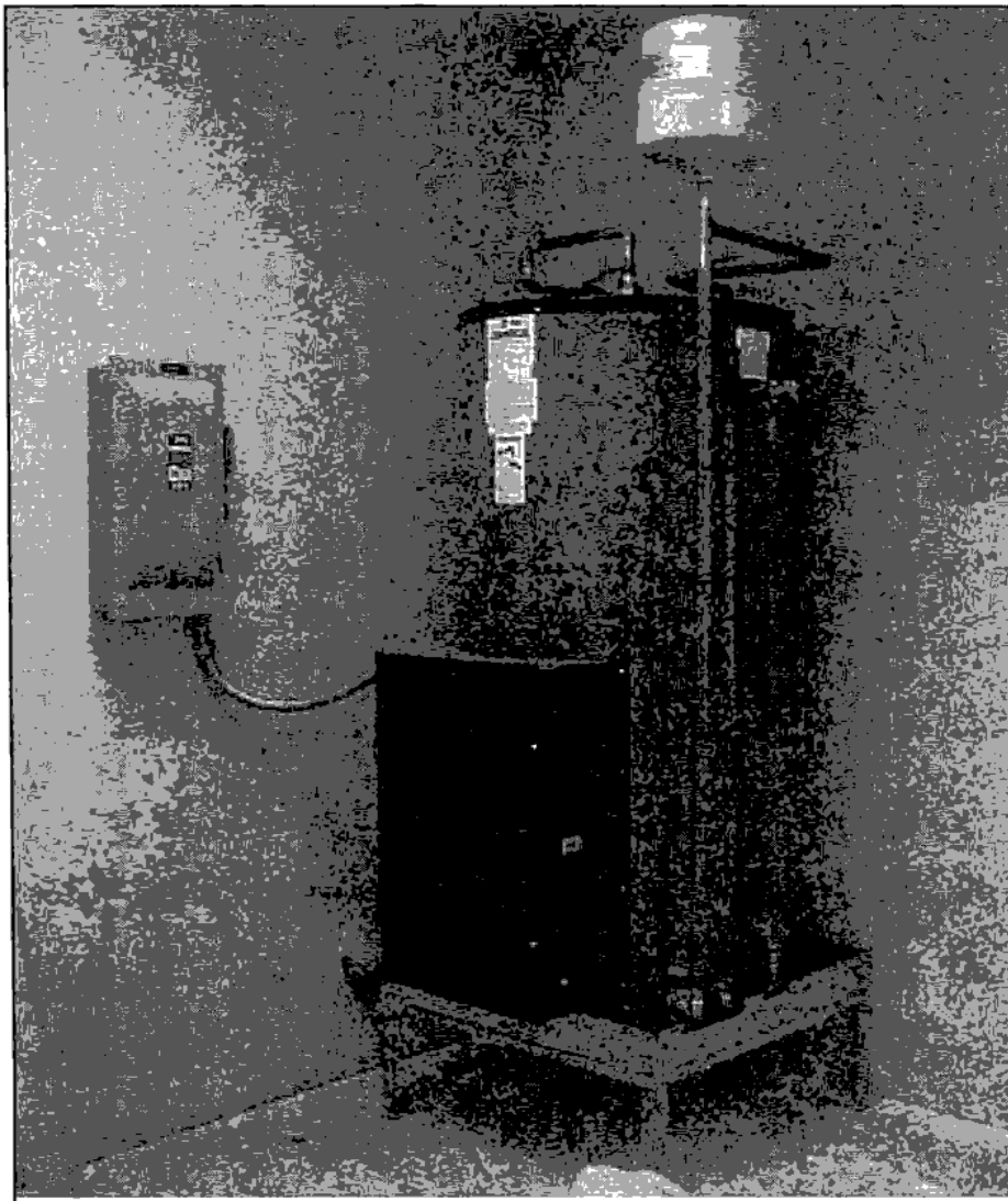
شکل (۴-۱۶-۵۹) قطع کن الکتریکی در مجاورت آب گرم کن
