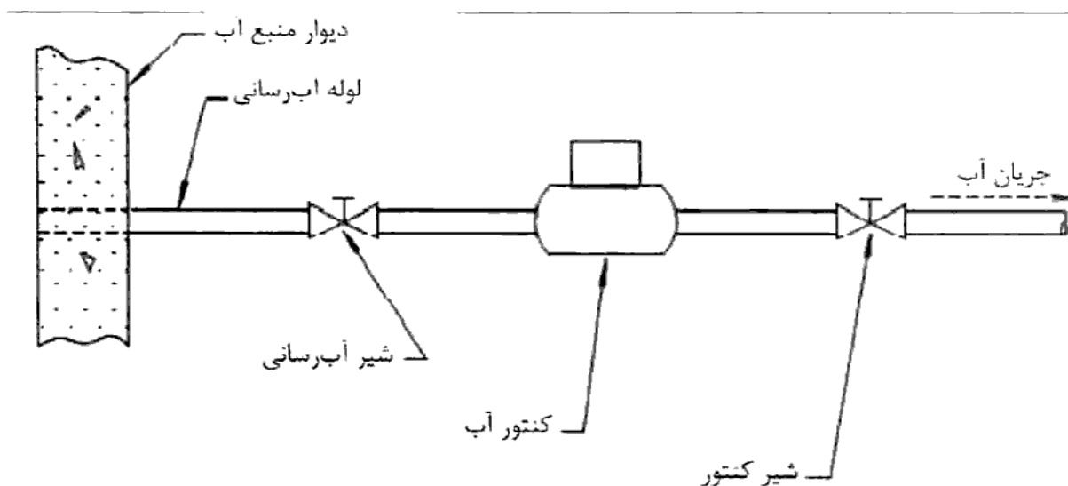
شکل (۱۶-۴-۱۵) شیر در ورودی ساختمان و در سمت تخلیه کنتور آب
