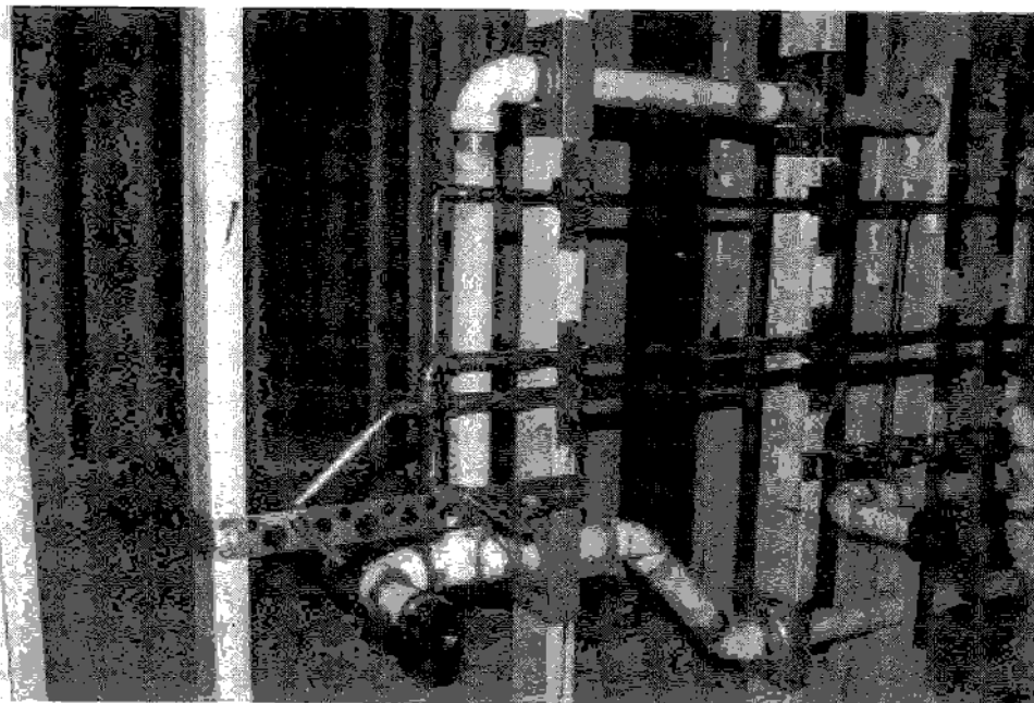
شکل (۱۶-۹-۱۴) بست‌های لوله‌های مسی افقی در محل اتصال به لوازم بهداشتی
