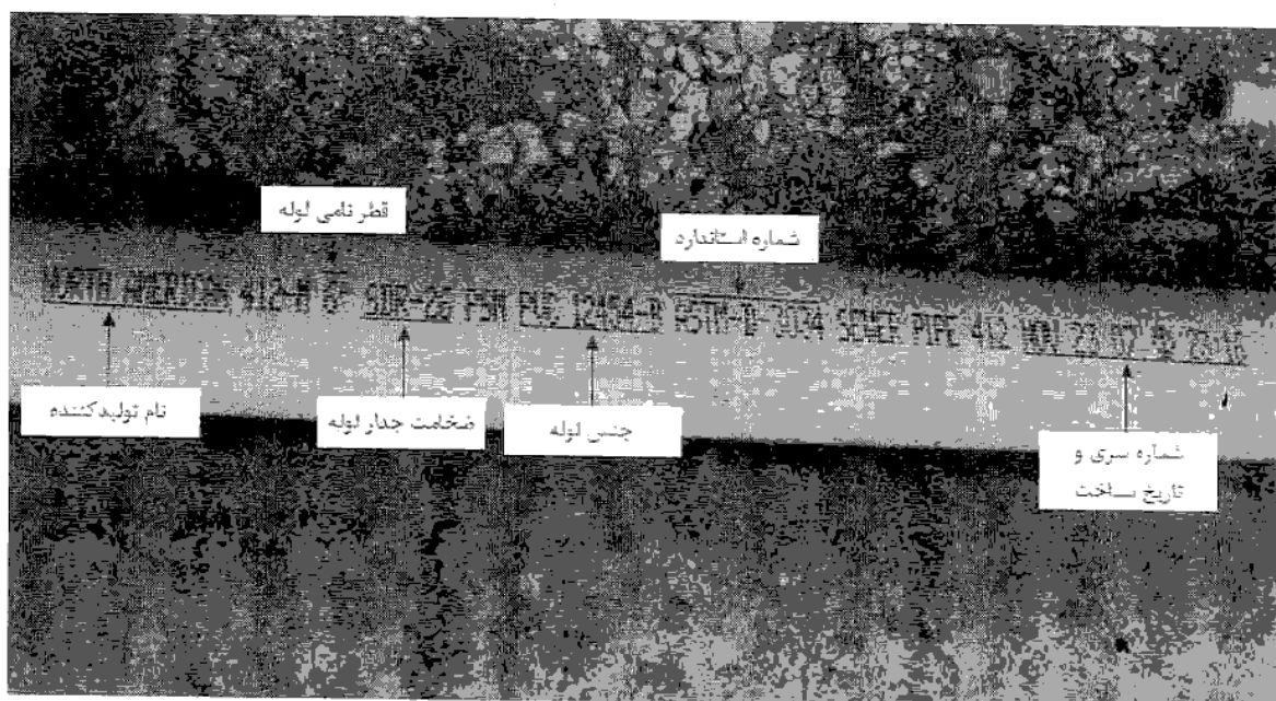
شکل (۱۶-۳-۱) نمونه‌ای از نحوه ثبت مشخصات بر روی لوله
