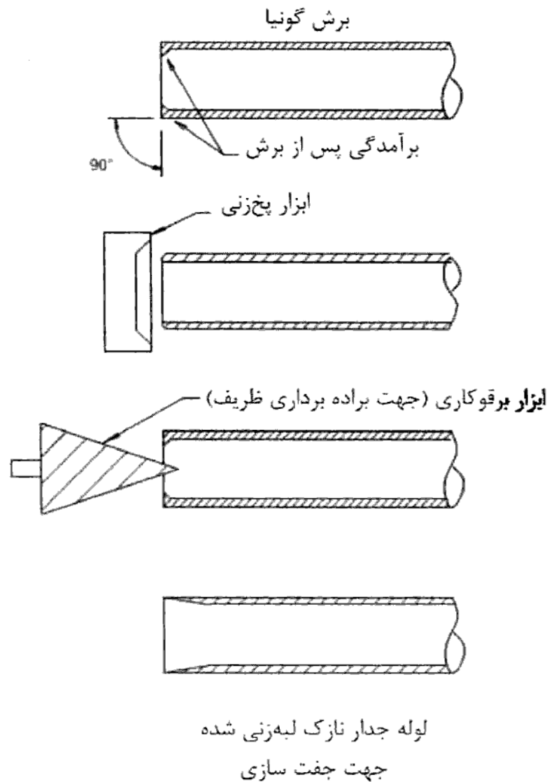
شکل (۷-۴-۱۶) آماده سازی انتهای لوله
