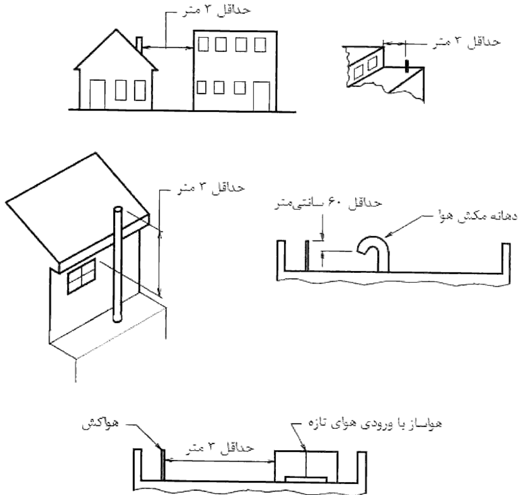
شکل شماره (۶-۶-۱۶) فاصله انتهایی هواکش عبوری از بام از بخش‌های مختلف ساختمان
