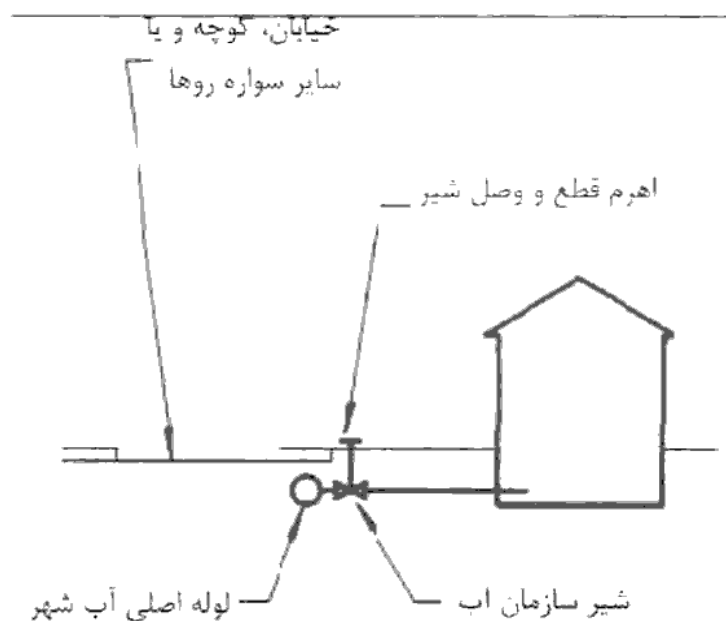
شکل (۱۶-۴-۱۴) شیر پیاده‌رو، بر روی لوله آبرسانی ساختمان
