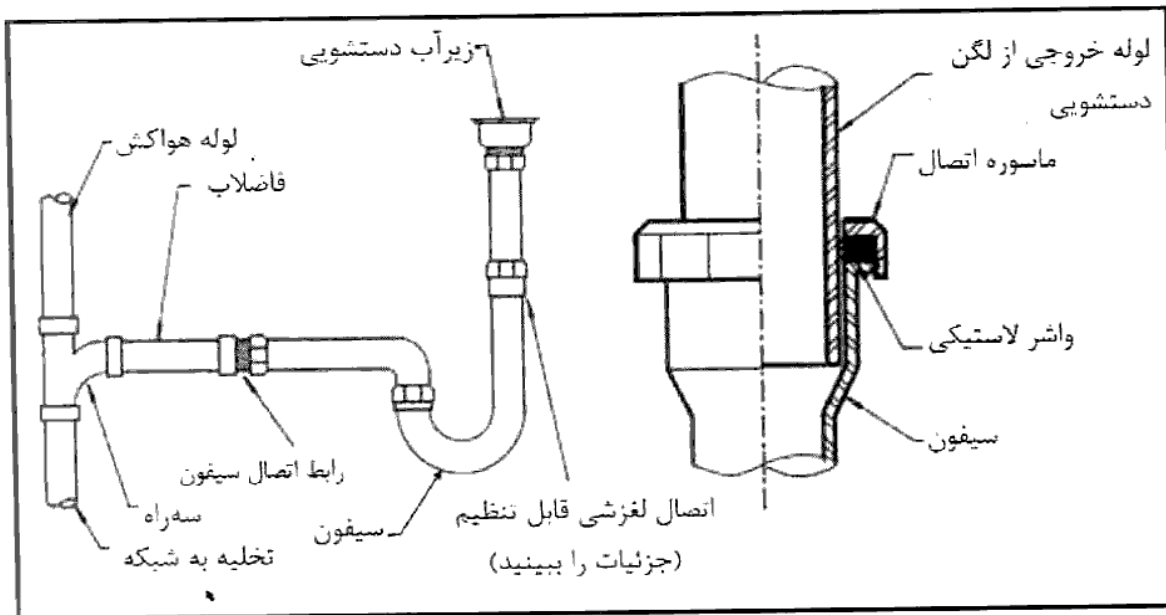
شکل (۱۶-۵-۵۰) اتصال لوله فاضلاب به لوازم بهداشتی
