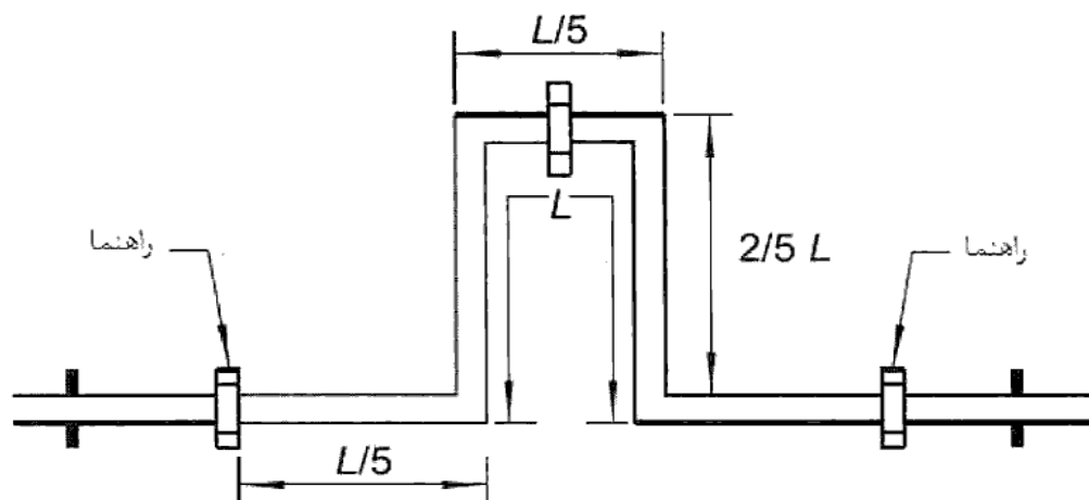
(پ) خم U شکل
