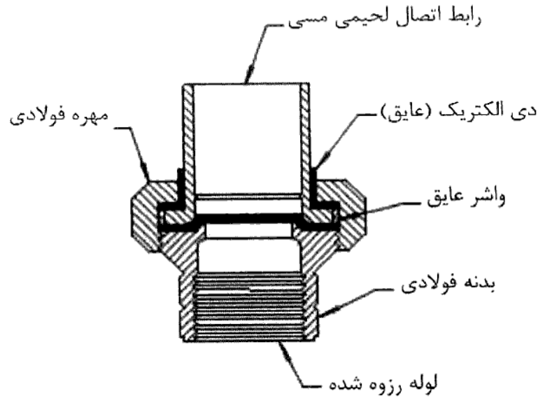
شکل (۱۱-۴-۱۶) مهره ماسوره دی الکتریک
