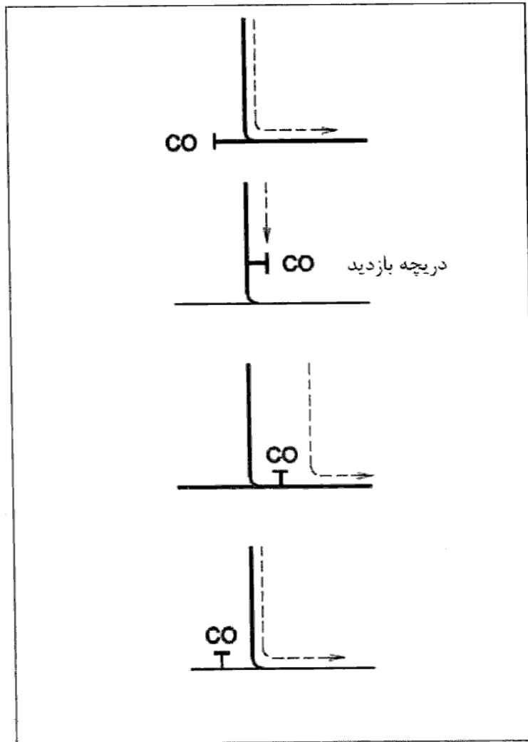
شکل (۱۶-۵-۱۵) دریچه بازدید در پائین لوله قائم
