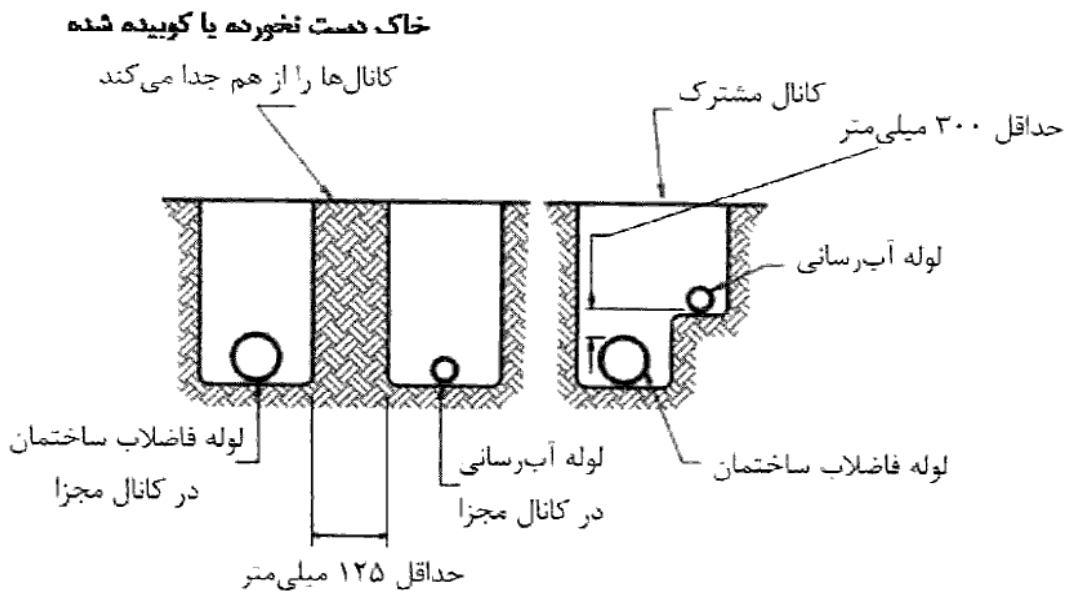
شکل (۴-۱۶-۴۴) کمینه فاصله بین لوله انشعاب اصلی و لوله فاضلاب ساختمان
