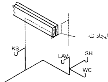
شکل شماره (۱۶-۶-۸) شیب لوله هواکش
