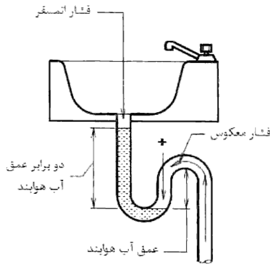
شکل شماره (۱-۶-۱۶) نحوه مقاومت آب هوا بند در برابر اختلاف فشار
