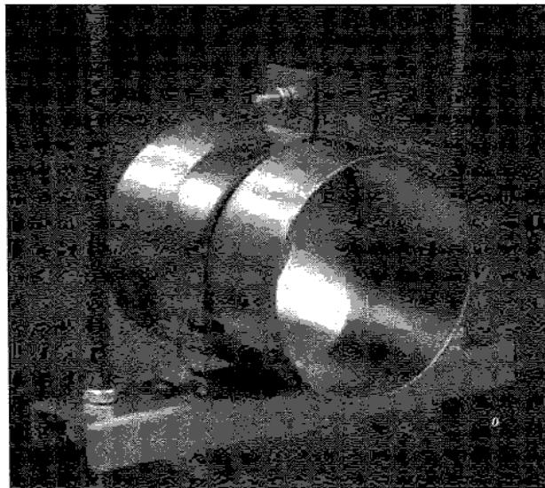
شکل (۱۶-۹-۱۳) بست و تکیه‌گاه فولادی گالوانیزه
