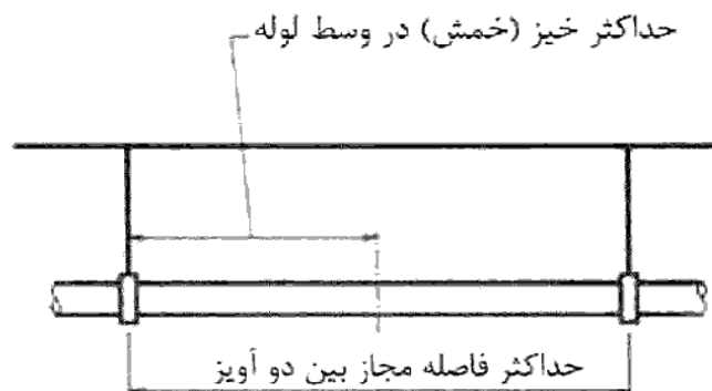
شکل (۱۶-۹-۱) موقعیت خمش بیشینه در بین دو آویز
