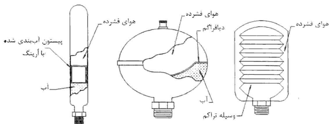
شکل (۱۶-۴-۲) نمونه‌هایی از وسایل مکانیکی حذف ضربه قوچ
