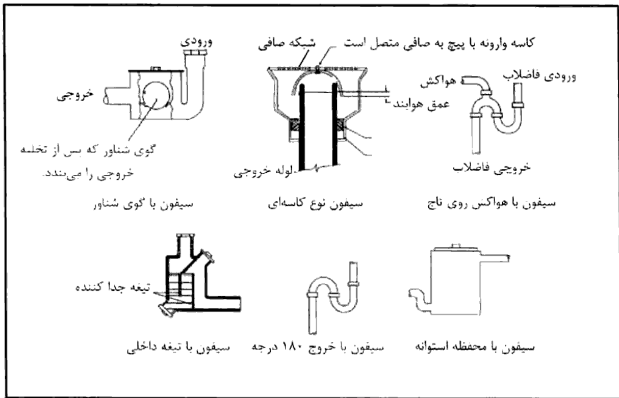
شکل (۱۶-۵-۳) انواع سیفون‌هایی که کاربرد آن‌ها ممنوع است
