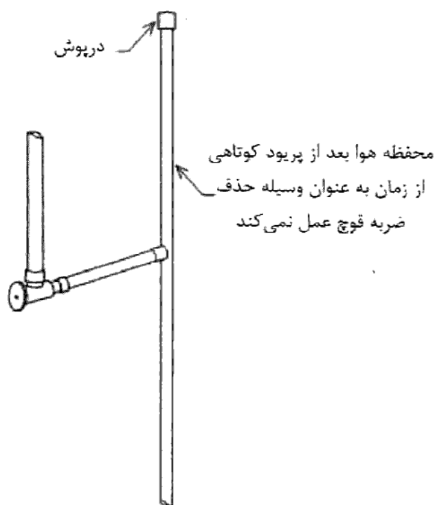
شکل (۱۶-۴-۳) وسیله حذف ضربه قوچ از نوع محفظه هوا
