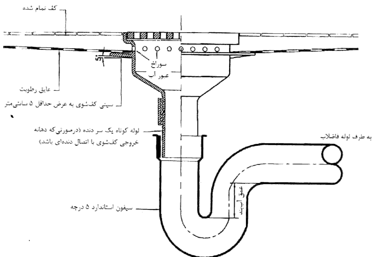
شکل شماره (۱۶-۷-۸) جزئیات نصب کفشوی با سیفون جدا
