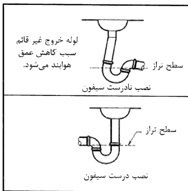
شکل (۱۶-۵-۵) چگونگی نصب سیفون
