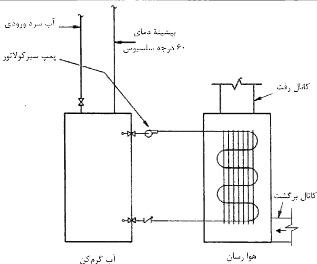
شکل (۴-۱۶-۴۶) مبدل حرارتی آب به هوا
