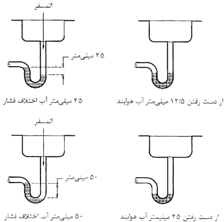
شکل شماره (۲-۶-۱۶) نحوه کم شدن عمق آب هوا بند بر اثر اختلاف فشار
