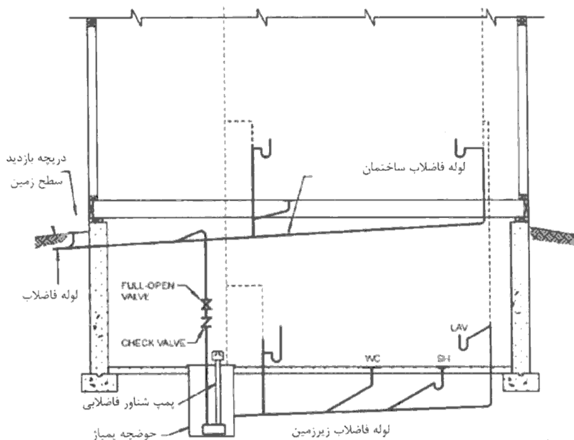
شکل (۱۶-۲-۸) استفاده از پمپ حوضچه فاضلاب برای انتقال فاضلاب به تراز بالاتر
