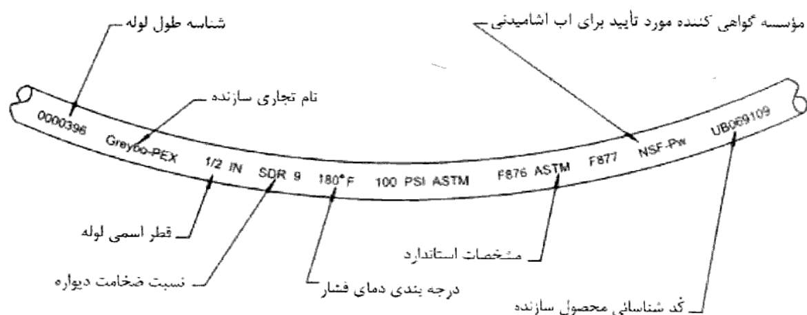
شکل (۱۶-۴-۶) نمونه‌ای از علامت‌گذاری روی لوله PEX
