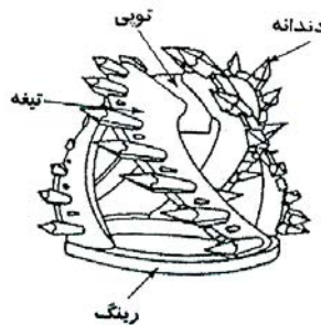
شکل ۵-۸-۷- انواع سر لایروب کاتراسکشن
