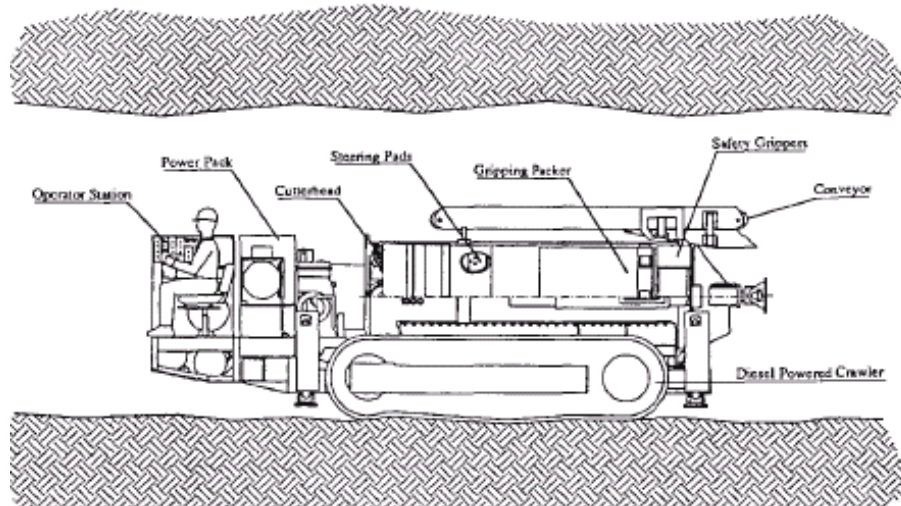
شکل ۳-۶-۲. نمائی از قابلیت حرکت ماشین در مقاطع کوچک
