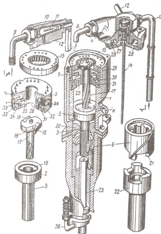
شکل ۳-۷-۱۸- اجزای پرفراتور
