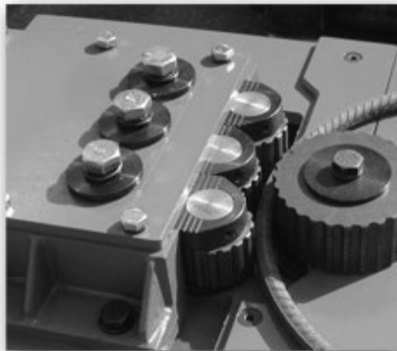
شکل ۴-۱۲-۱۲- ماشین خم میلگرد به فرمهای فنری و اسپیرال
