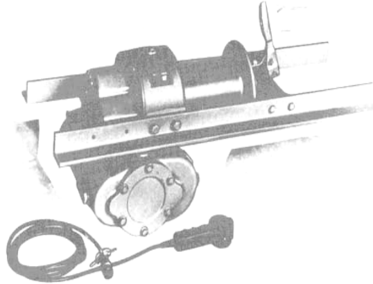
شکل ۶-۹-۴- وینچ الکتریکی
