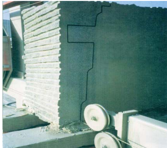
شکل ۳-۱۷-۳- ایجاد شکل‌های مختلف روی سنگ با استفاده از سیم برش
