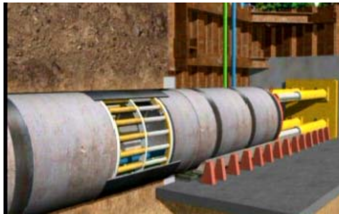
شکل ۵-۱۰-۹- ایستگاه جک های میانی
