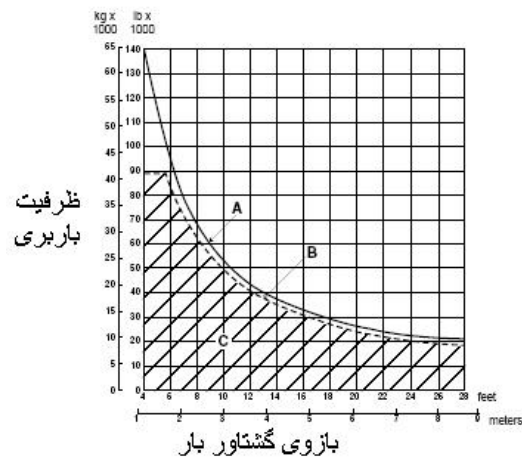
نمودار ۳-۱-۵ - نمودار ظرفیت باربری مدل ۵۸۳R
