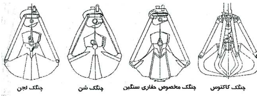
شکل ۵-۸-۱۰- جام لایروب پانتون چنگی
