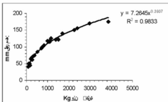
شکل ۳-۱۰-۱۷- اثر وزن چکش بر قطر سرمته
