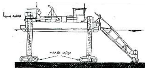
الف : نوع خرنده با بوری سره برش افقی تخلیه بیهیا بوری خرنده
