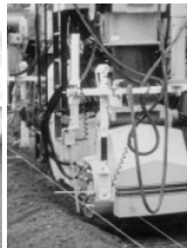
شکل ۴-۱۶-۱۱- کنترل مسیر بوسیله ریسمان و یا به صورت الکترونیکی (دو روش مختلف)
