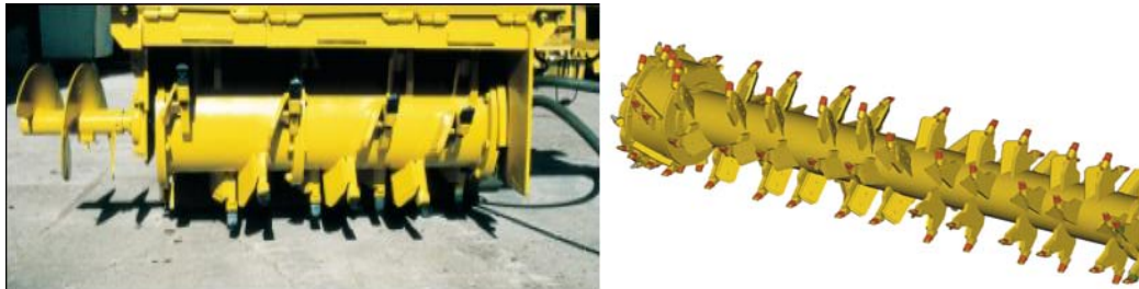
شکل ۲-۱۸-۷- تریمر هد
