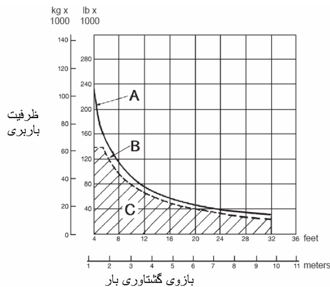
نمودار ۴-۱-۵ - نمودار ظرفیت باربری مدل ۵۸۹
