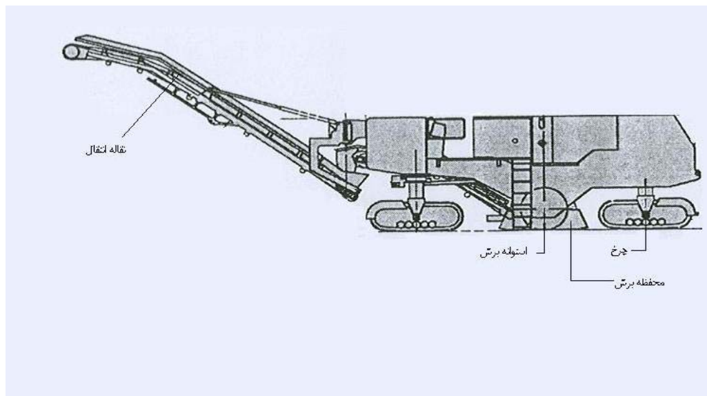
شکل شماره ۲-۱۳-۴- قسمت‌های مختلف ماشین‌آلات تراش
