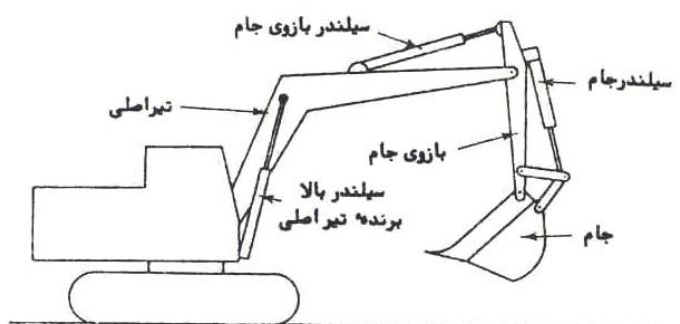
شکل ۲-۱۰-۳- قسمت های مختلف بیل هیدرولیکی جام معکوس
