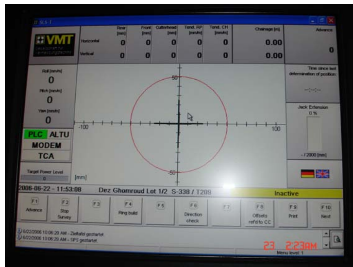
شکل ۳-۳-۳۶. صفحه اصلی نشاندهنده حرکت دستگاه در راستای مورد نظر که میزان انحراف را از مسیر که با ردیاب لیزری کنترل می‌شود، مشخص می‌کند.
