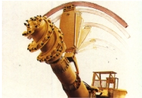
شکل ۳-۱۶-۷- ماشین رودهدر به همراه تجهیزات نصب قاب
