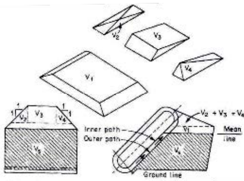
شکل ۲-۶-۹- اسکرپرهای نقاله‌دار و تعیین ظرفیت آنها
