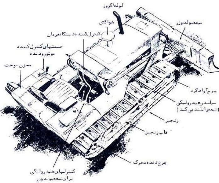
شکل ۶-۱-۵- تراکتور چرخ زنجیری
