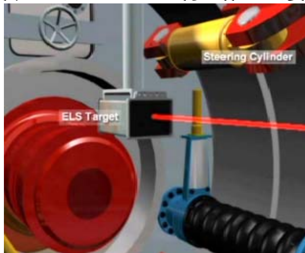
شکل ۹-۶-۱۵- کنترل مسیر توسط اشعه لیزر
