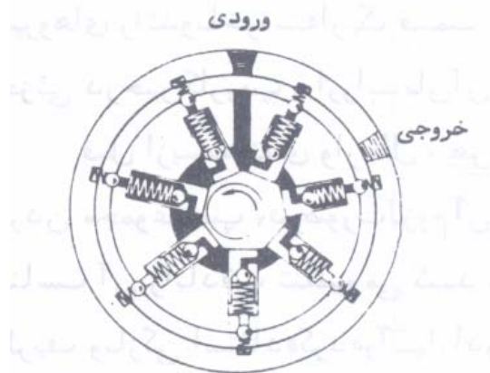
شکل ۶-۱۱-۱۰- نحوه کار پمپ پرده‌ای پیستونی
