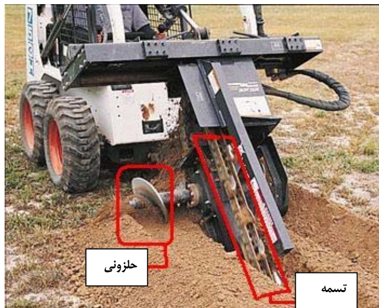
شکل ۲-۱۵-۴- قسمت‌های اصلی نهر کن
