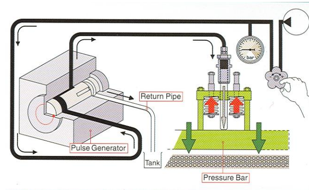
شکل شماره ۲-۸-۱۹- اهرم فشار
